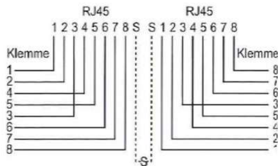
Schéma de la prise c8
